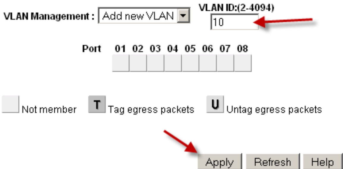
Fig. 105: Add VLAN 10
