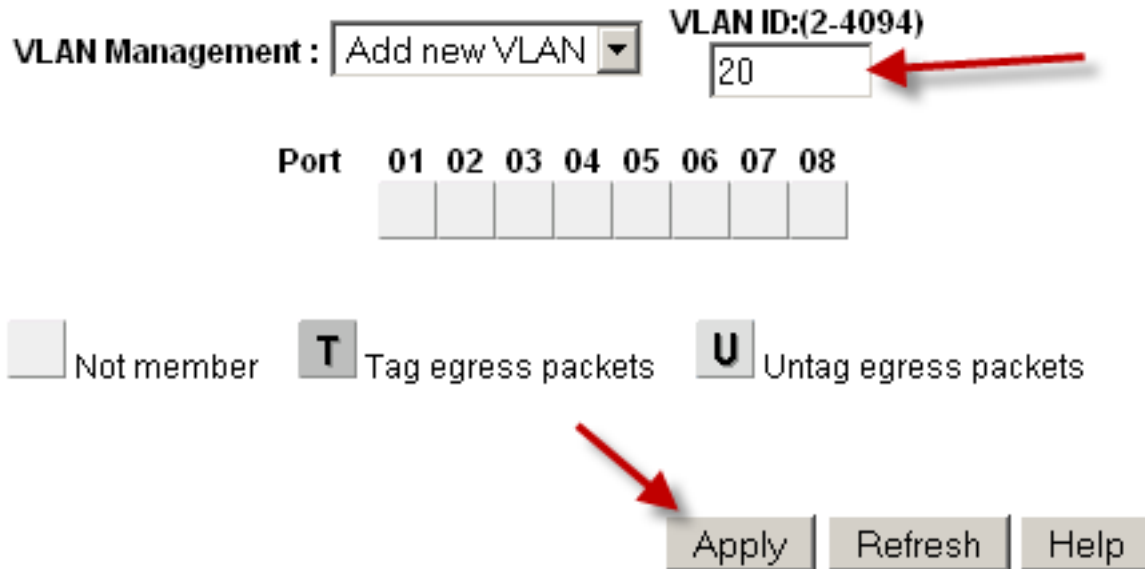
Fig. 106: Add VLAN 20
